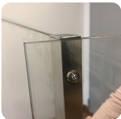
Sujeción con taladros
